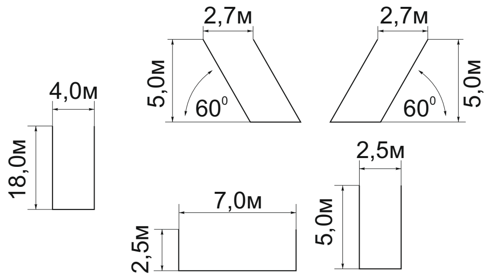
Размеры стояночного места
