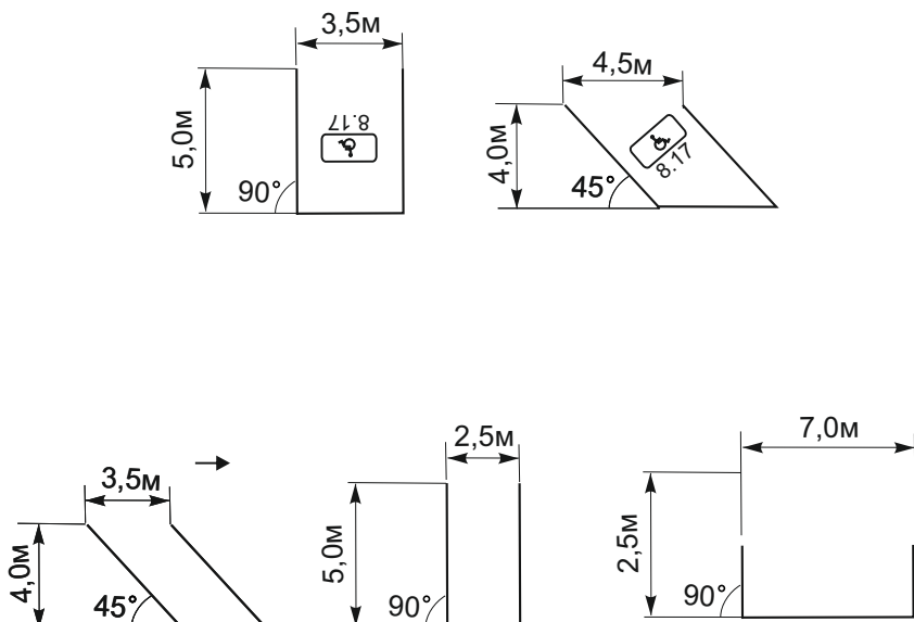
Размеры стояночных мест
